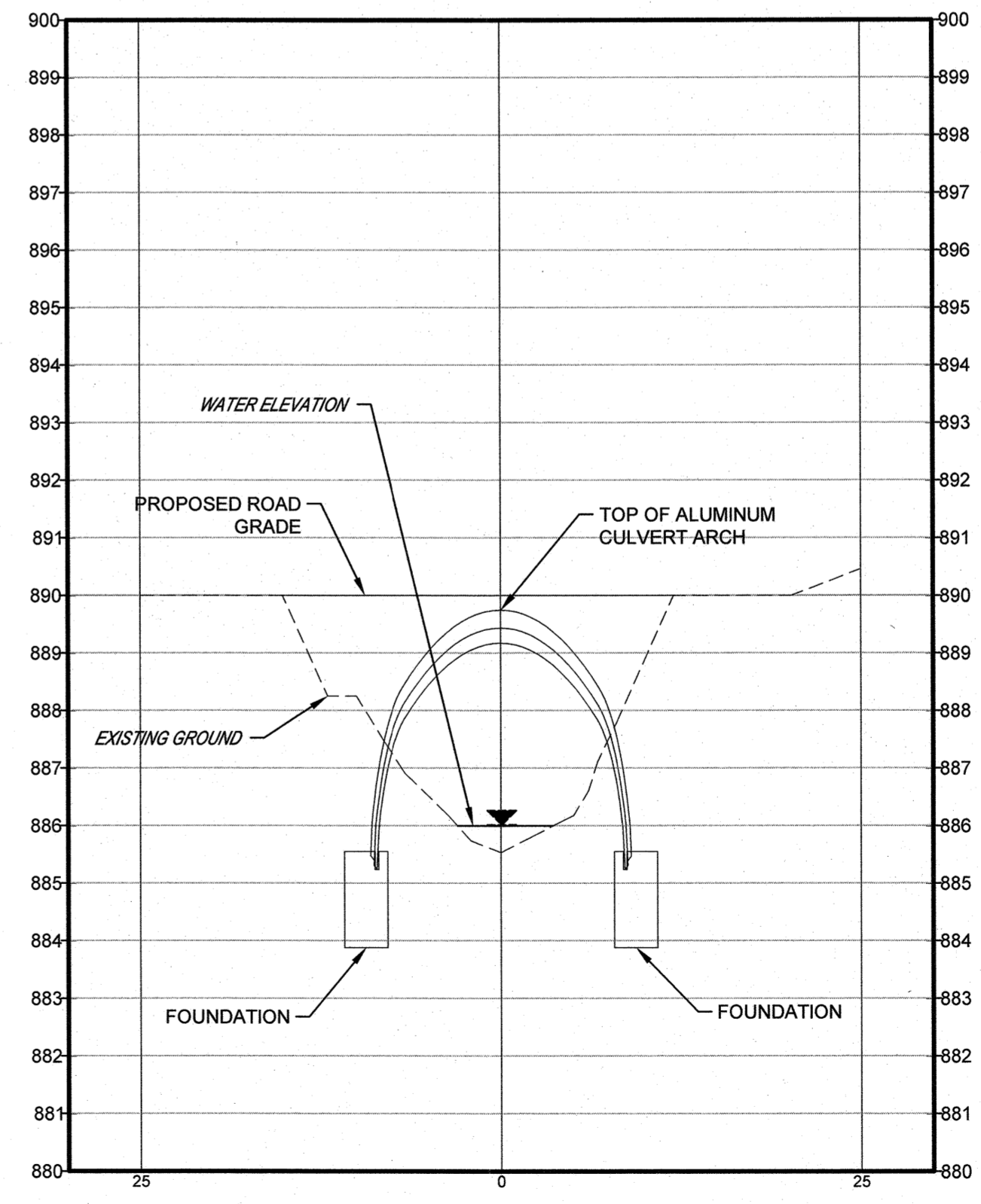
SECTION B HORIZONTAL SCALE: 1" = 10' VERTICAL SCALE: 1" = 2.5'
