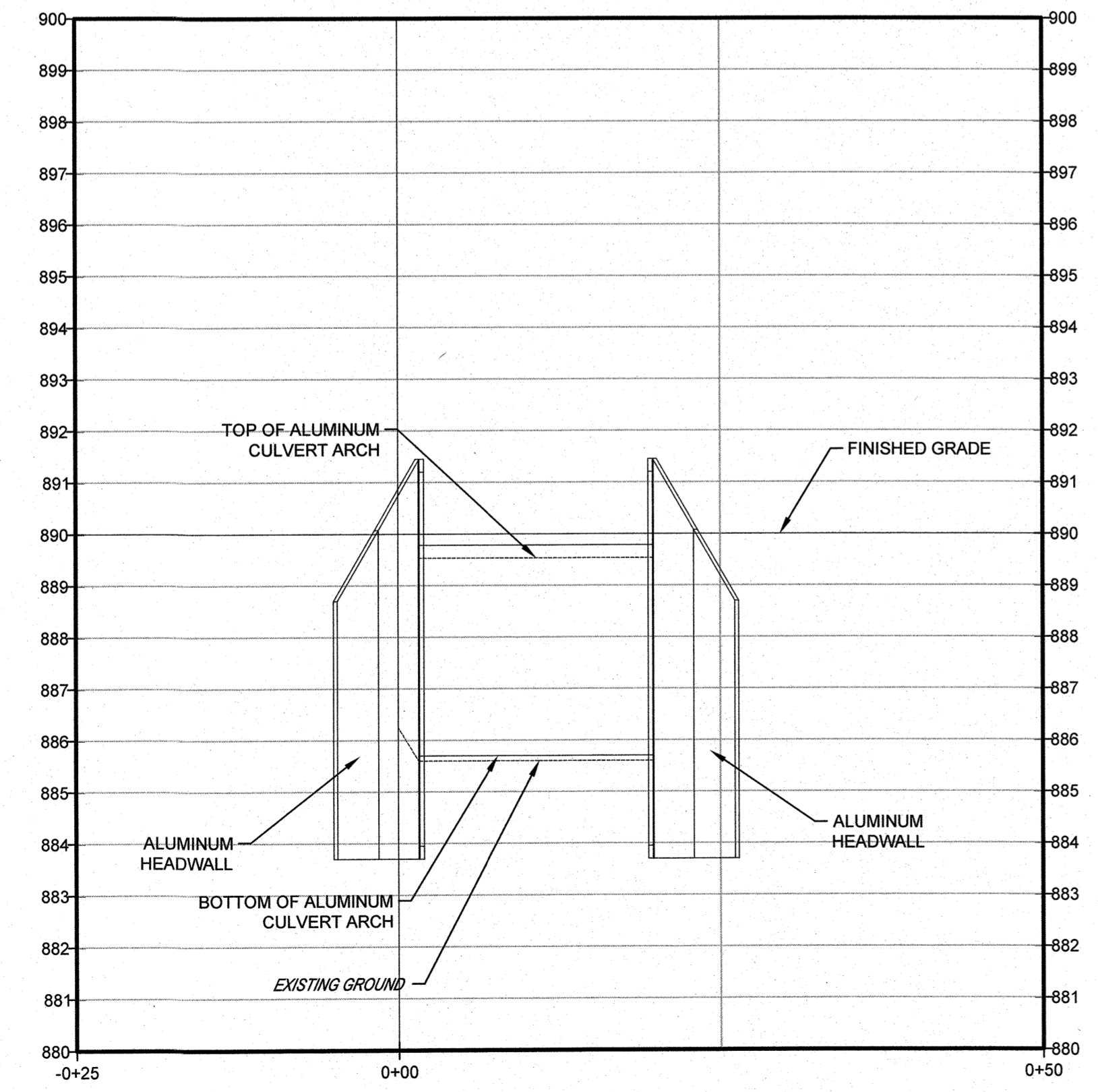
SECTION A HORIZONTAL SCALE: 1" = 10' VERTICAL SCALE: 1" = 2.5'
